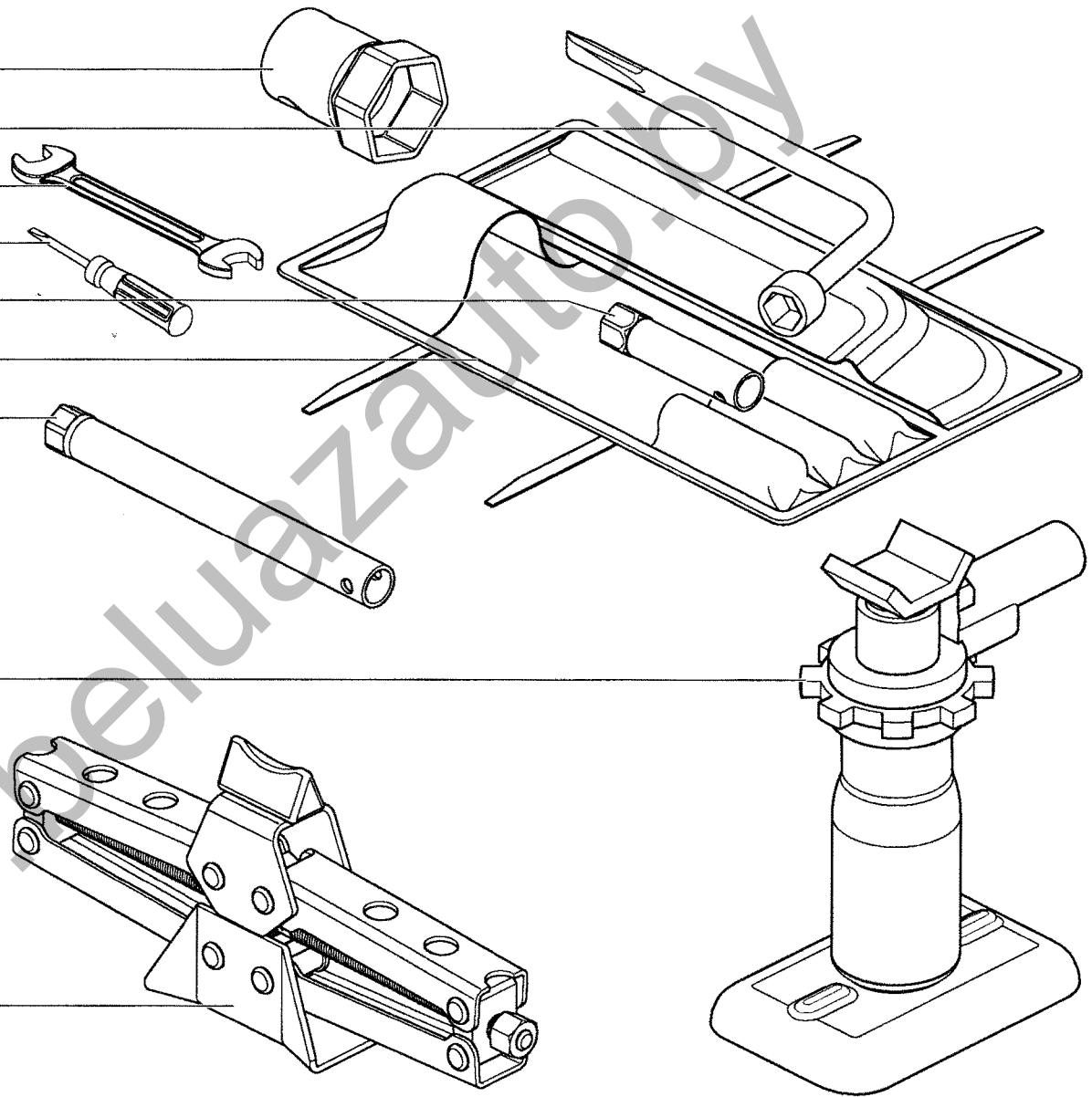
Рис. 143. Инструмент водителя и принадлежности (3901), домкрат (3913) Fig. 143. Driver's tools and accessories (3901), jack (3913)
