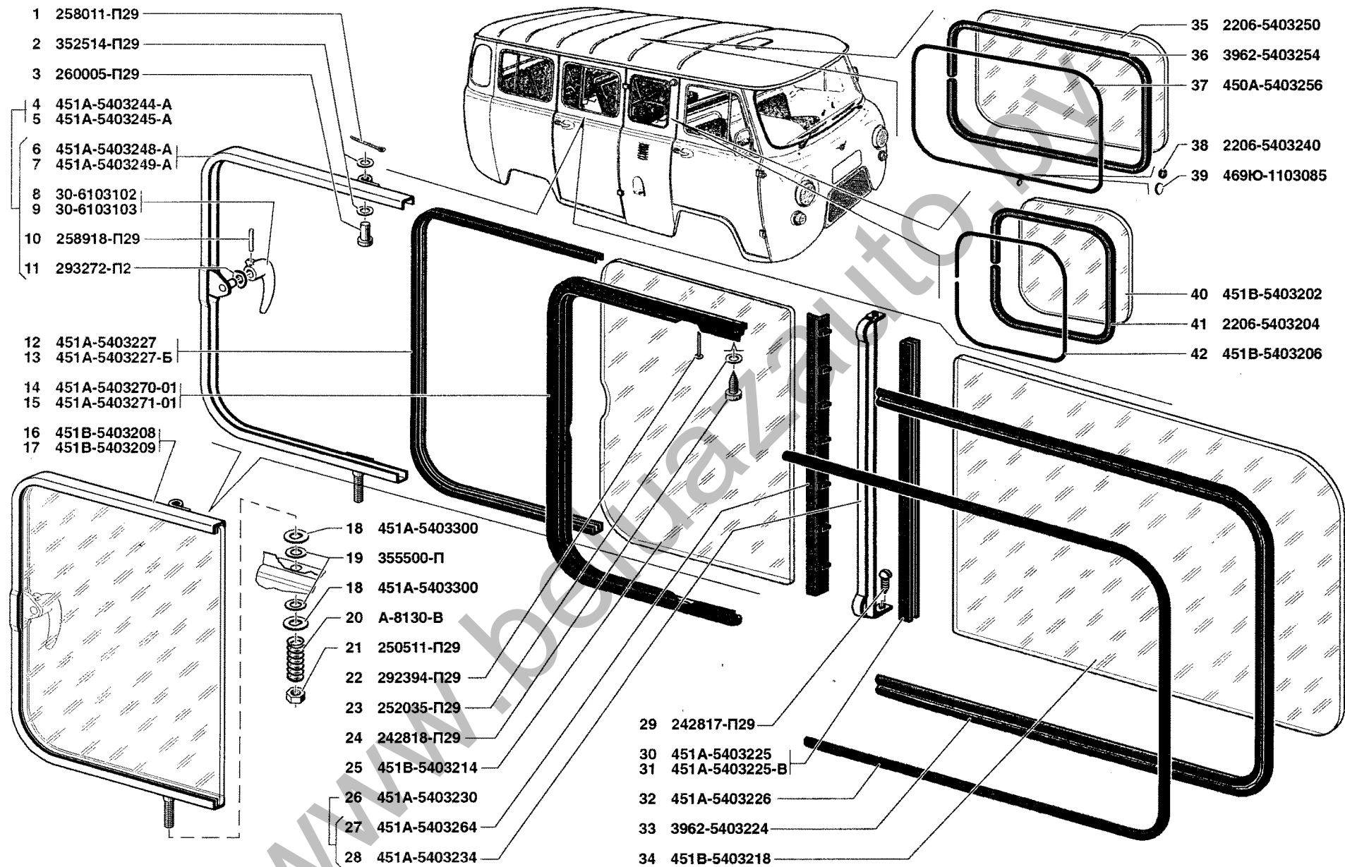
Рис. 153. Окно боковины поворотное (5403) Fig. 153. Body side swivelling window (5403)
