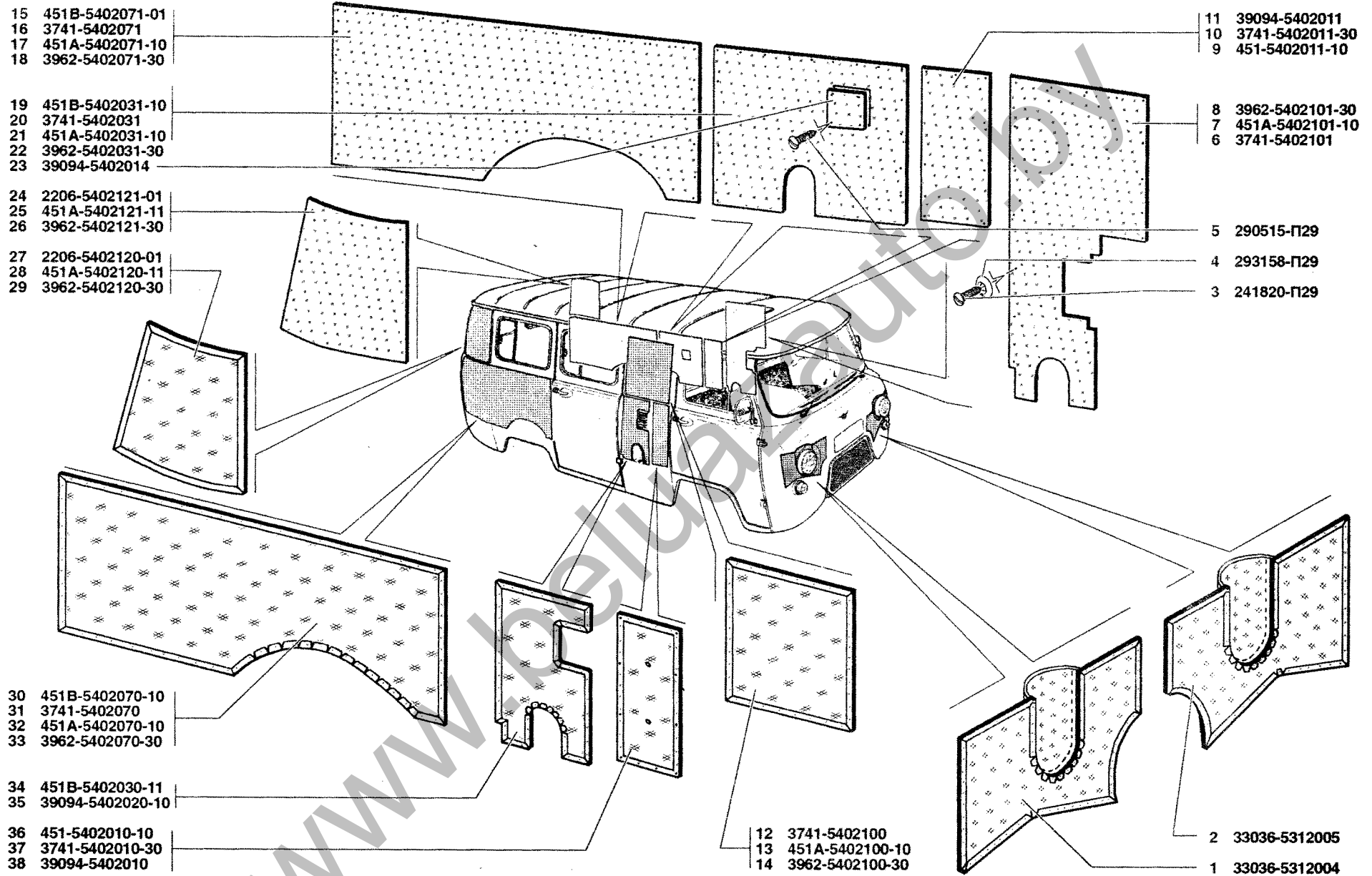
Рис. 152. Термозвукоизоляция передка (5312), обивка боковины (5402) Fig. 152. Body front sound-and-heat insulation (5312), body side lining (5402)
