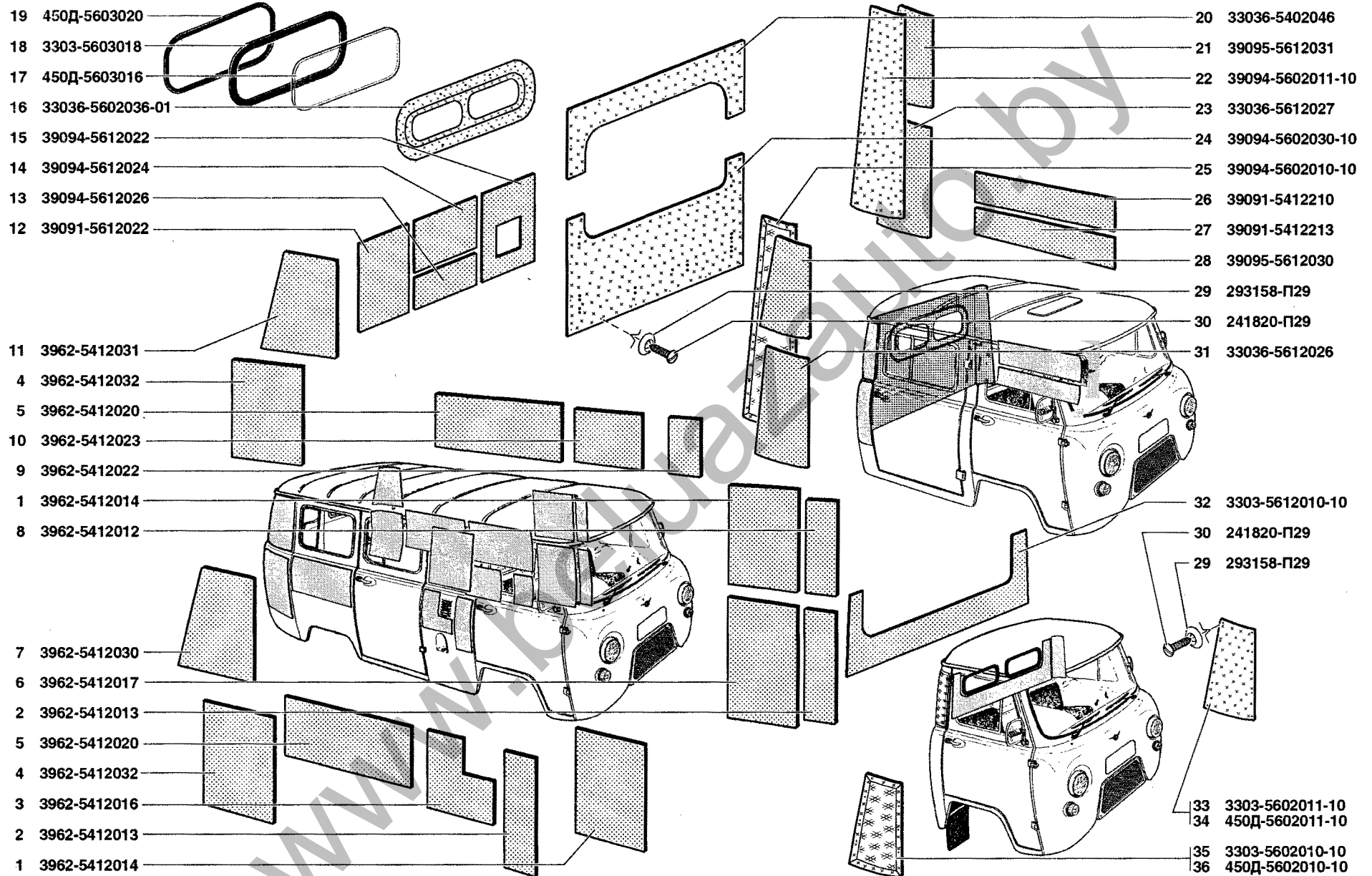
Рис. 154. Термошумоизоляция боковины (5412), обивка задка (5602), окно задка (5603) Fig. 154. Side panel sound-and-heat insulation (5412), body rear lining (5602), body rear window (5603)
